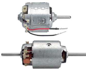
Motor de eletrôventilador interno
