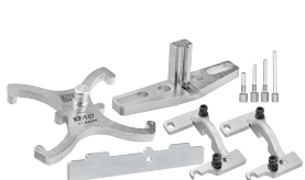
KF-162 KIT SÍNCR. COMANDO DE VÁLV. MOTOR FORD KA 1.0 3CIL TI-VCT 14>16 1.5 16V SIGMA 14>15 FIESTA 1.0 3CIL ECOBOOST 11>16 1.5 16V SIGMA 11>13
