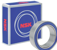
38BD5417 38X54X17 10P08 GOL PARATI PALIO SIENA
