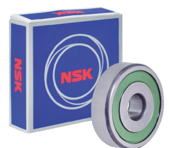
B17-126DDWC3 17X62X17,5
