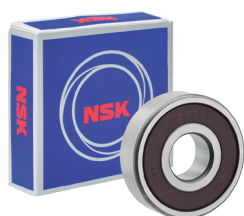
6303DDUC3 17X47X14
