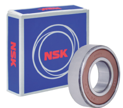
6205DDU 25X52X15
