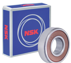
6204DDUC3 20X47X14
